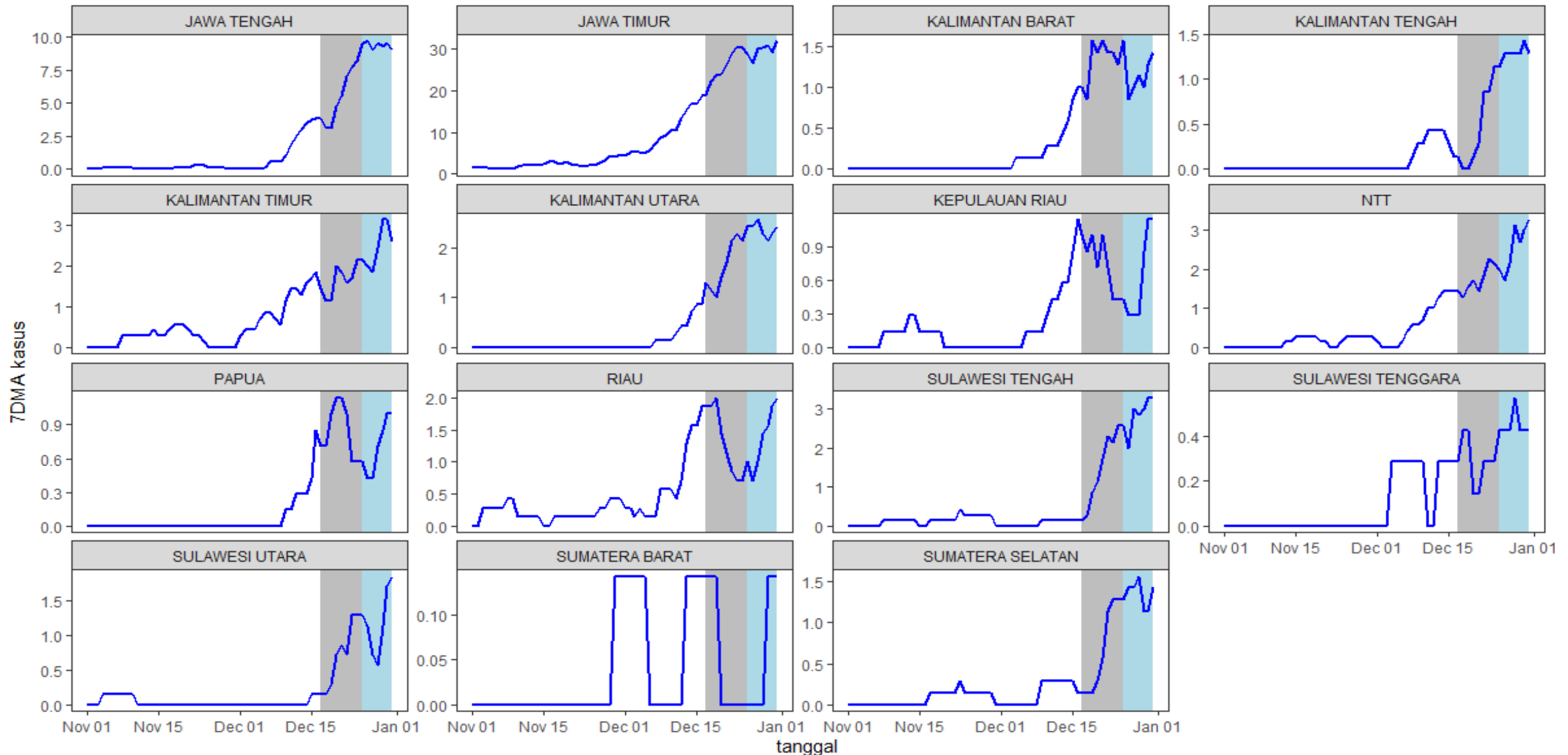
Trend 7DMA Kasus Harian Yang Meningkat dibandingkan Minggu Sebelumnya (per 31 Desember 2023 )
